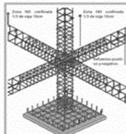
6_Armado Viga
